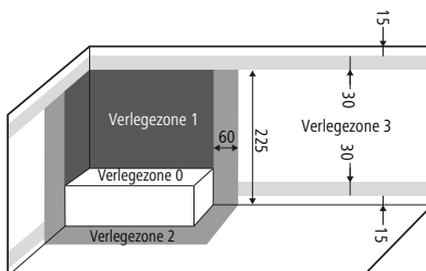
Abb. 1: Verlegezone
