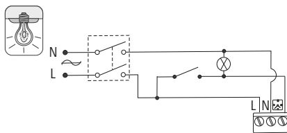
Abb. 4: Verdrahtung mit extern geschaltetem Steuermodul - Schaltbild
