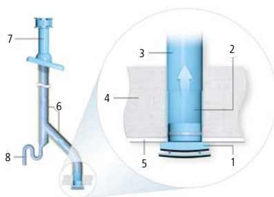
Abb. 7: Deckenmontage
