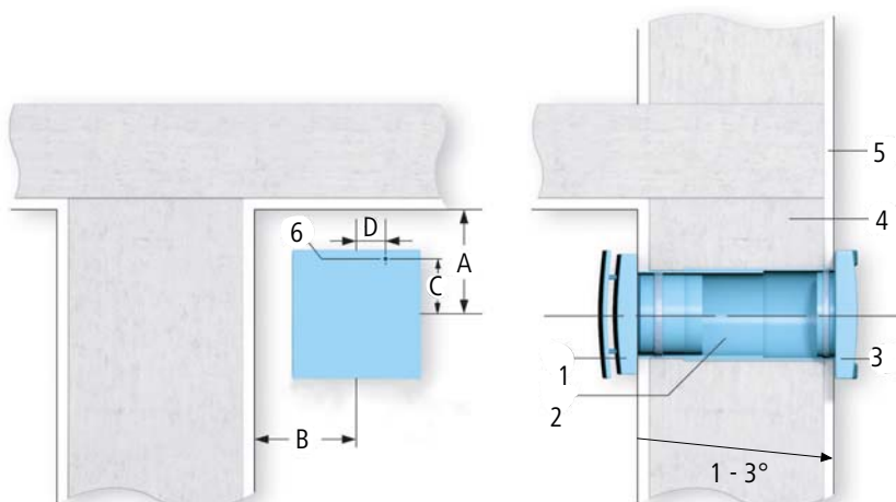
Abb. 3: Wanddurchbruch
