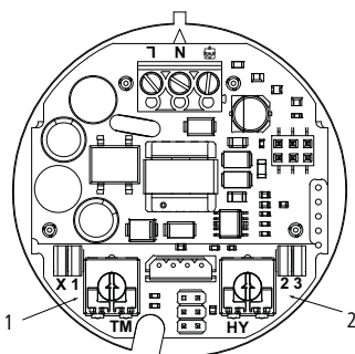
Abb. 6: Trimmereinstellung
